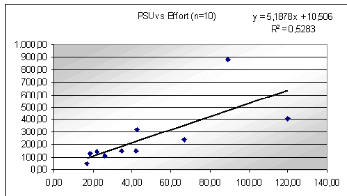
Fig. 14 – Conjunto de Datos de N=10 proyectos y ecuación de regresión lineal (R 2 =52.83%)
