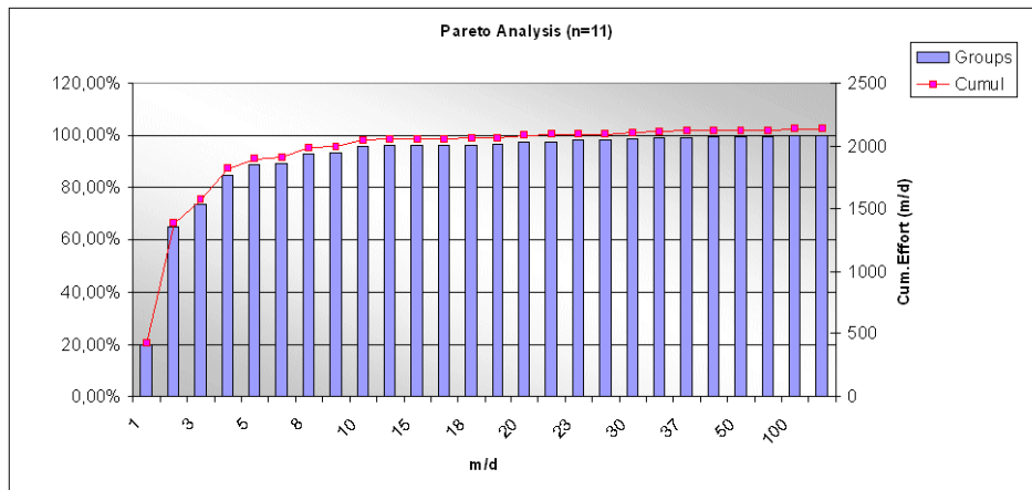
Fig. 12 –Análisis de Pareto (Histograma) con 11 proyectos
