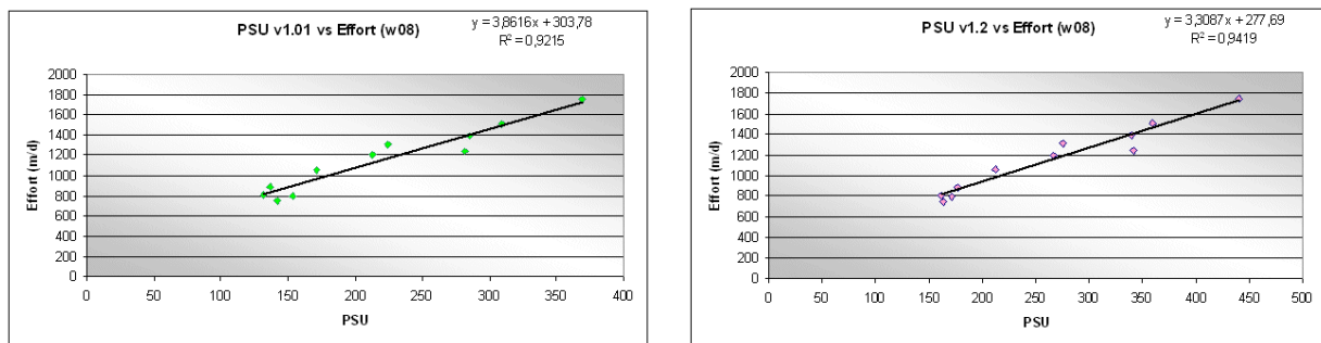
Fig. 9 – PSU vs Esfuerzo (n=11): versión 1.01 y versión 1.2
