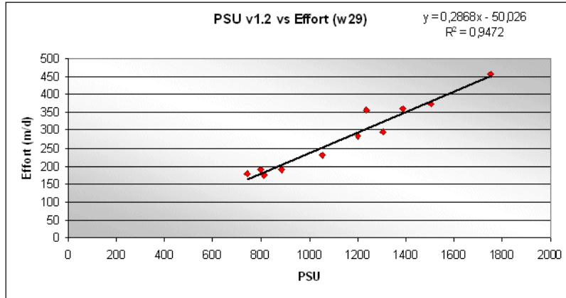
Fig. 13 – Evaluación con los nuevos pesos de tareas (w.29)
